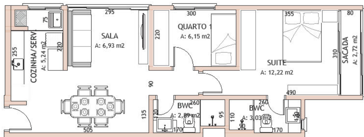
APARTAMENTO TIPO 5 A: 58,20 m2
