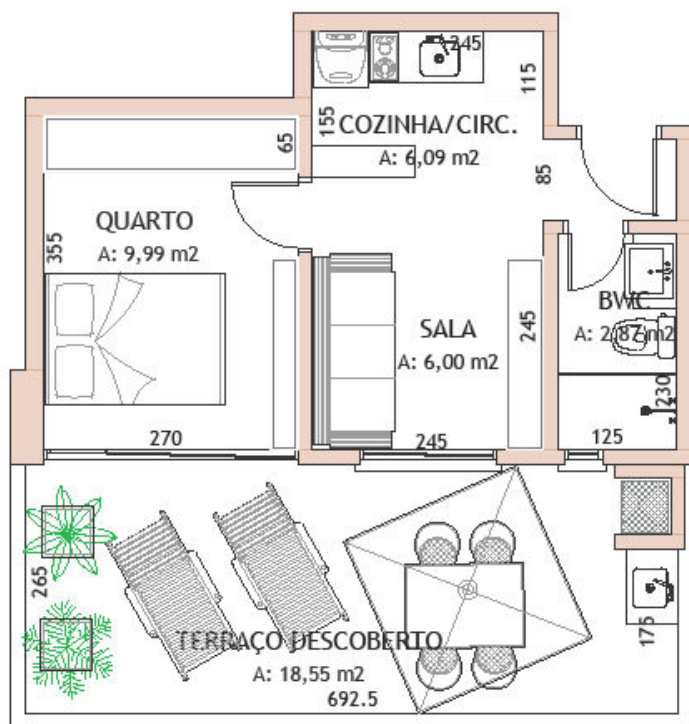
ESTUDIO GARDEN A: 29,02 m 2
