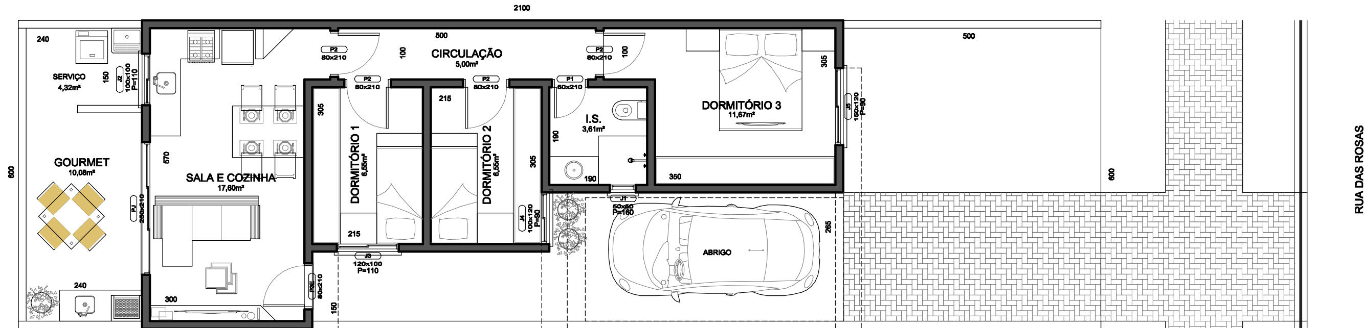
PLANTA BAIXA A=59,59m²
